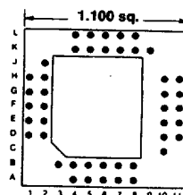
44 PINS Footprint 11041
