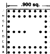
55 PINS Footprint 09010
