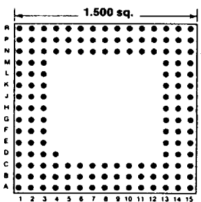
145 PINS Footprint 15024
