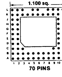
Footprint 11028
