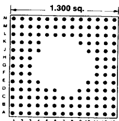
133 PINS Footprint 13048
