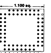
64 PINS Footprint 11040
