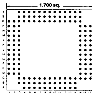
145 PINS Footprint 17004
