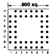
44 PINS Footprint 08003
