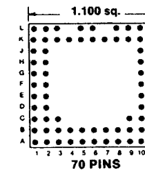
Footprint 11028
