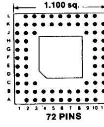
Footprint 11026
