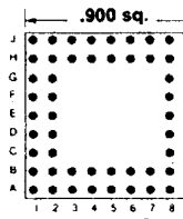
56 PINS Footprint 09009
