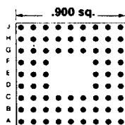
72 PINS Footprint 09004
