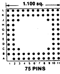
Footprint 11016
