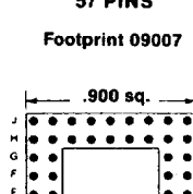
56 PINS Footprint 09008
