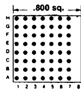
56 PINS Footprint 08004
