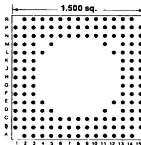
149 PINS Footprint 15019
